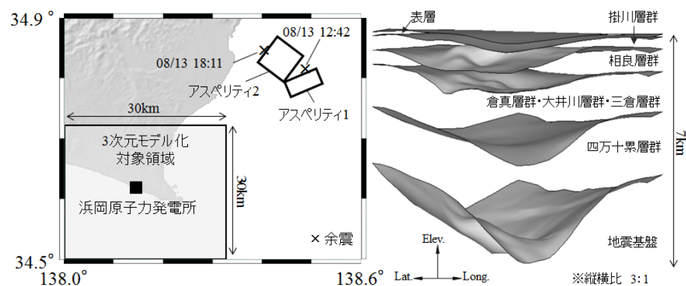
図1 2009年駿河湾の地震の3次元強震動シミュレーションに用いた震源モデル 1) と浜岡発電所周辺における深層および浅層の3次元地下構造モデル
